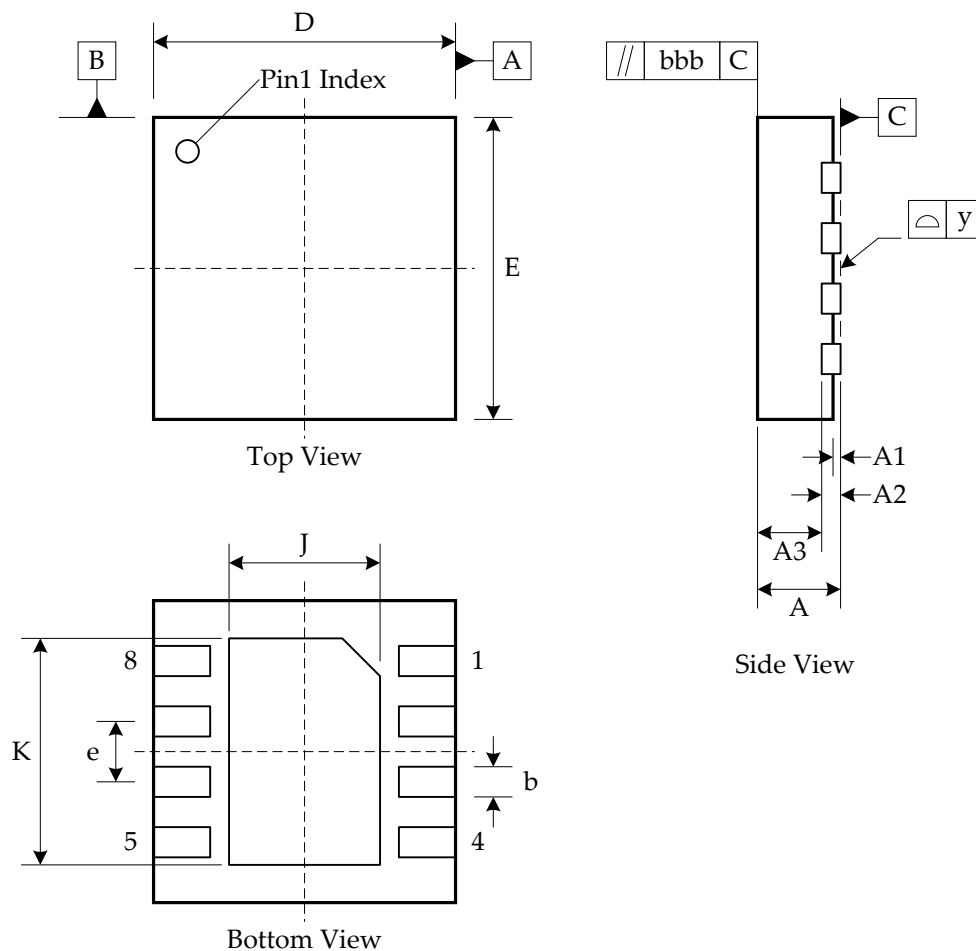
Figure 47: USON8(4*4mm) Package
